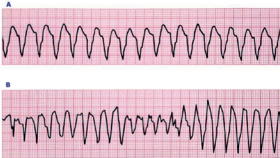
شکل ۱۹. تاکی کاردی بطنی (VT)، A. VT در کودک مبتلا به دیستروفی عضلانی و کاردیومیوپاتی شناخته شده. B. Torsades de B. pointes در کودک مبتلا به هیپومینیزیمی.
